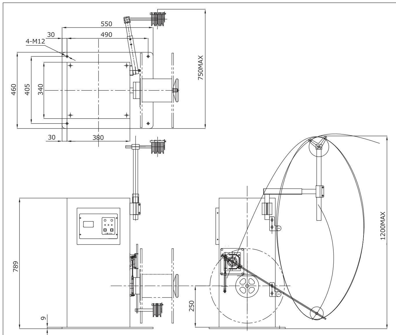
外形図
